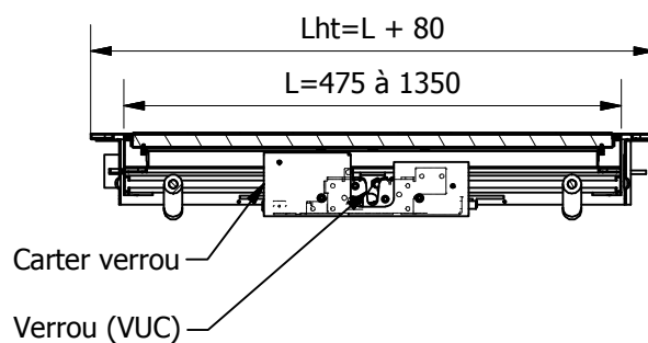
A-A ( 1/10 )
